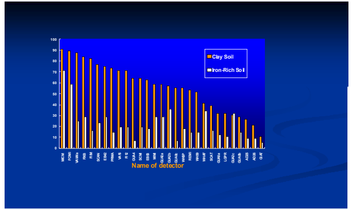
Şekil 7. Farklı yapıdaki metal dedektörlerin killi ve demirce zengin topraklardaki patlayıcıları bulma yüzdesini gösteren grafik
